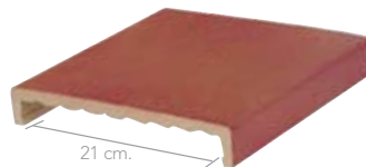
Pasamanos 21 x 24,5 x 4 cm 8,2" x 9,6" x 1,5" Ref. PAS 211
