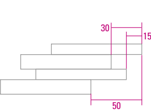
Modulo a due formati 15x90 (57,7%) - 11x90 (42,3%) fuga minima 2 mm.
