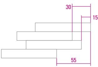
Modulo irregolare a un formato fuga minima 2 mm.
