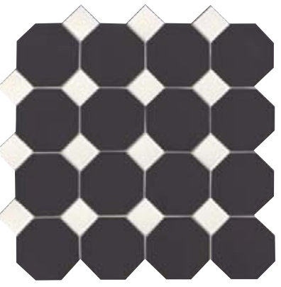
1m² ENMALLADO (G 52) compuesto por: 68 piezas CAPRICE OCTG.-5 12,2 x 12,2 68 piezas TACO CAPRICE 5 x 5
