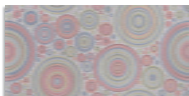
Geo Arena G.76
