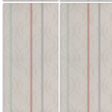
Gramínea - 6 Arena G.61
