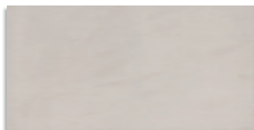
Cuarcita-R Arena G.174
