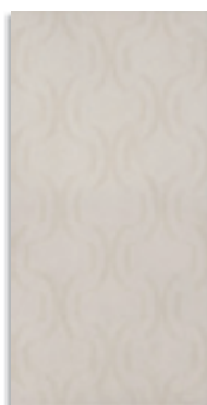
Turmalina Arena G.175
